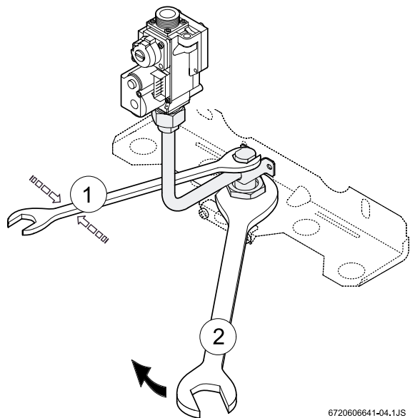
Fig. 8 Collegamento gas
