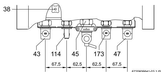
Fig. 6 piastra d'allacciamento
