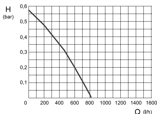
Fig. 4 Curva caratteristica del circolatore
