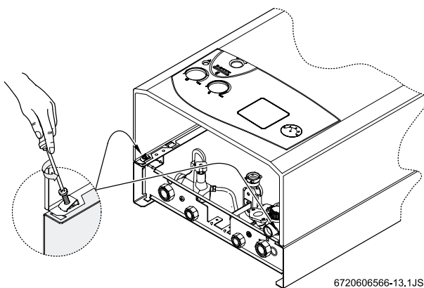
Fig. 7 Mantello
